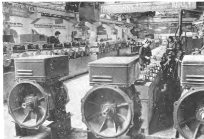
Երևանի Վ. Ի. Լենինի անվան «Հուլիսյան հեղեղ» գործարանի գեներատորների արտադրամասը:
